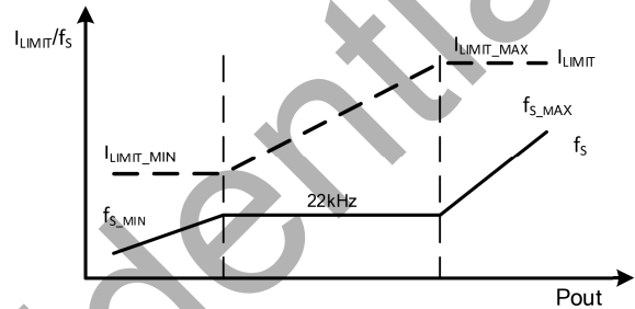
图 8. 控制模式
