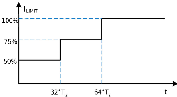
图 6. 软启动过程
