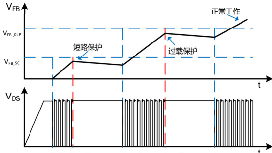
图 9. 短路保护、过载保护工作模式
