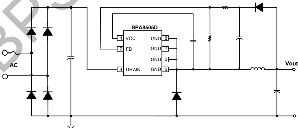
图 1. BPA8505D 典型 Buck 应用电路
