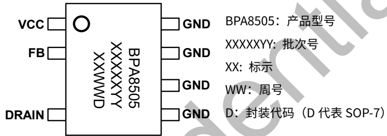
图 2. SOP-7 管脚封装图
